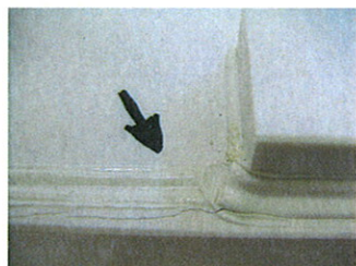
写真1：亀裂部拡大
