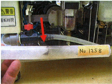
写真1:排水シリコンチューブ
