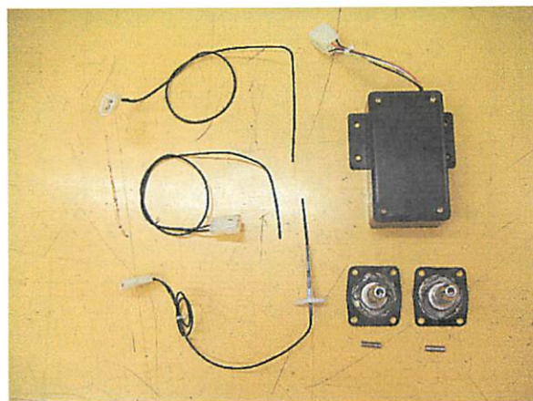
写真3：水位センサー、オゾンセンサー、給水電磁弁ダイヤフラム
