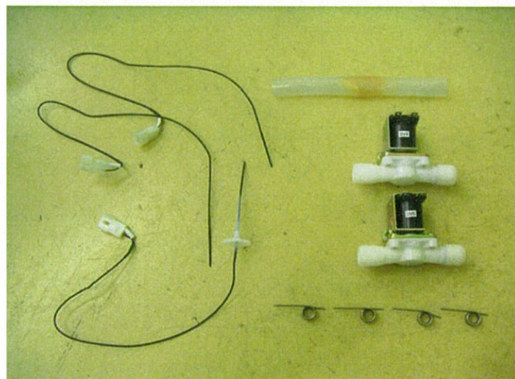
3 : 水位レベルセンサー、給水電磁弁、フタスプリング、排水バルブ用チューブ
